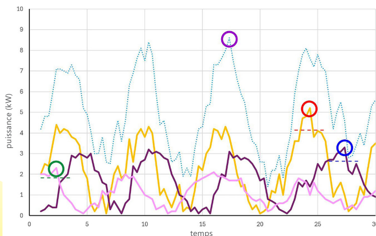
Courbes de puissance par compteur et total (1 mois)
